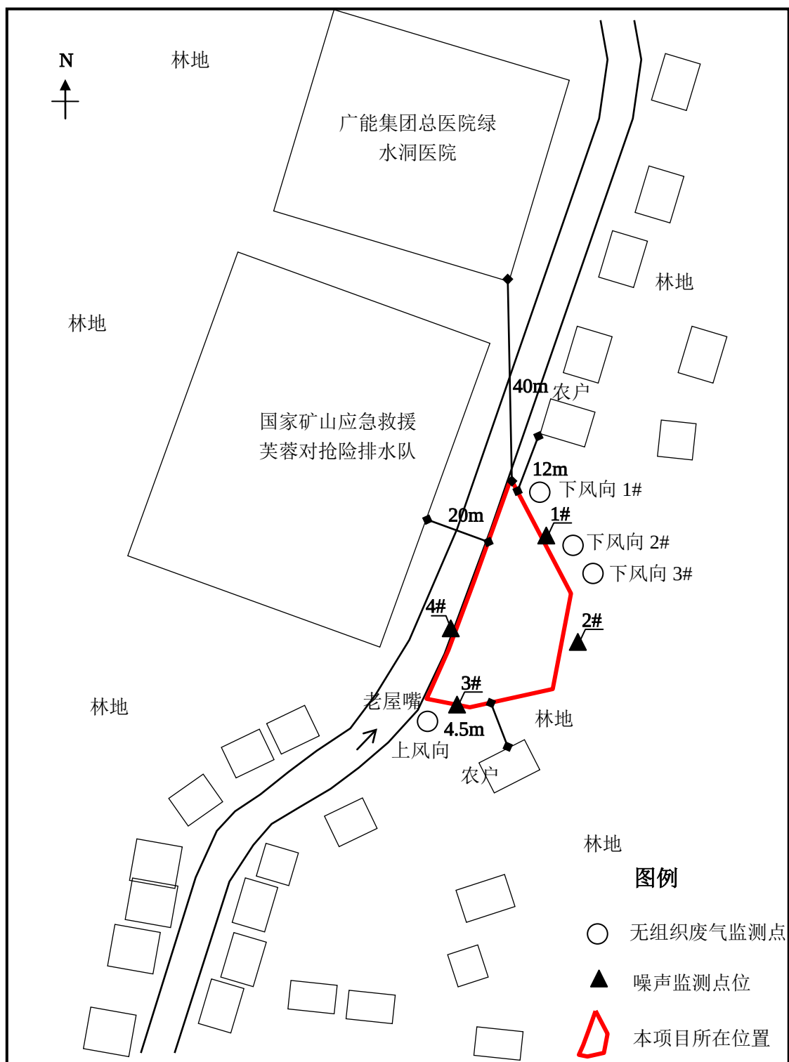
附图3 项目外环境关系及监测布点图
