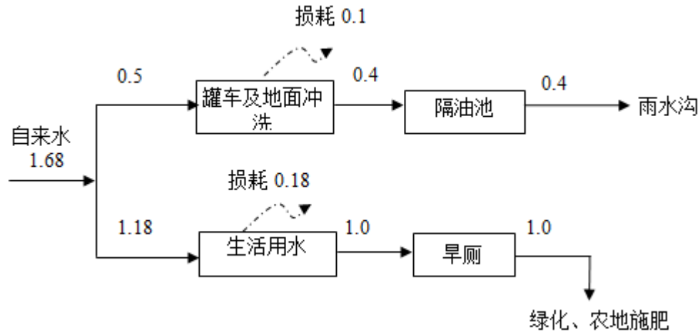
图 2-1 项目水平衡图 (消耗单位: m³/d)
